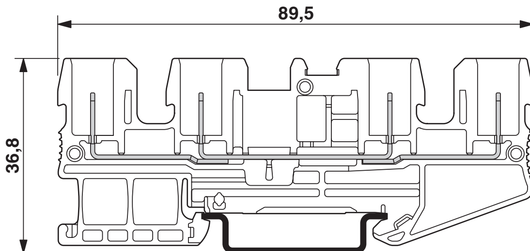
Måttskiss
