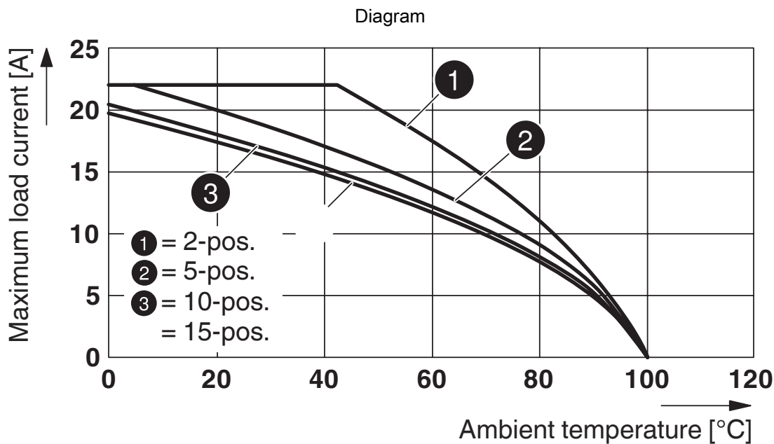
Deratingkurva för STTB 2,5/ 2P, STTB 2,5/ 2P-PV och för alla kontaktvarianter SP...
