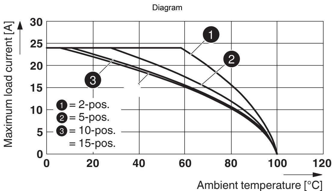
Deratingkurva för ST 2,5-QUATTRO/2P, ST 2,5-QUATTRO/4P och för alla kontaktvarianter SP...
