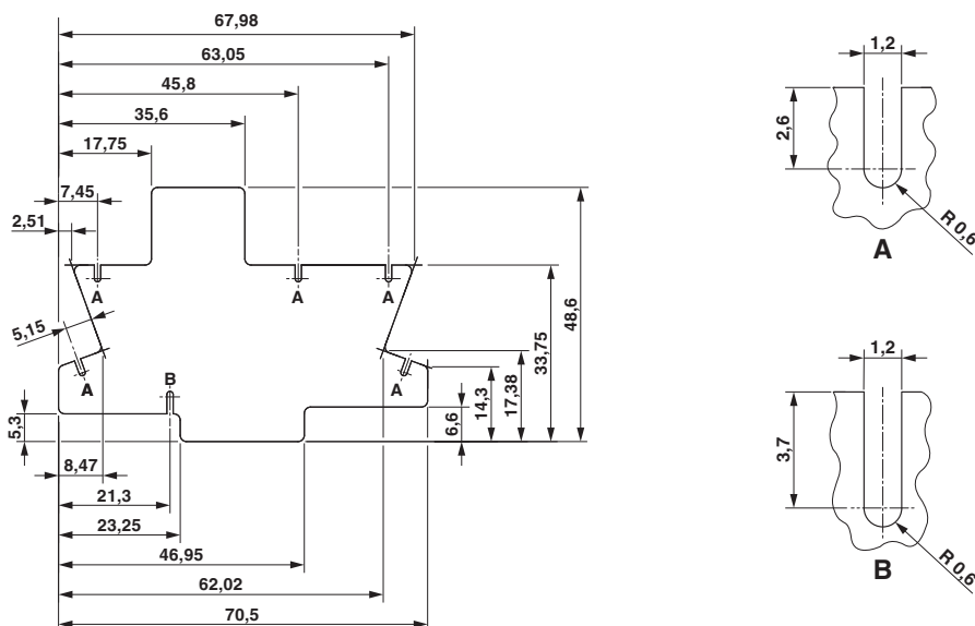
Måttskiss
