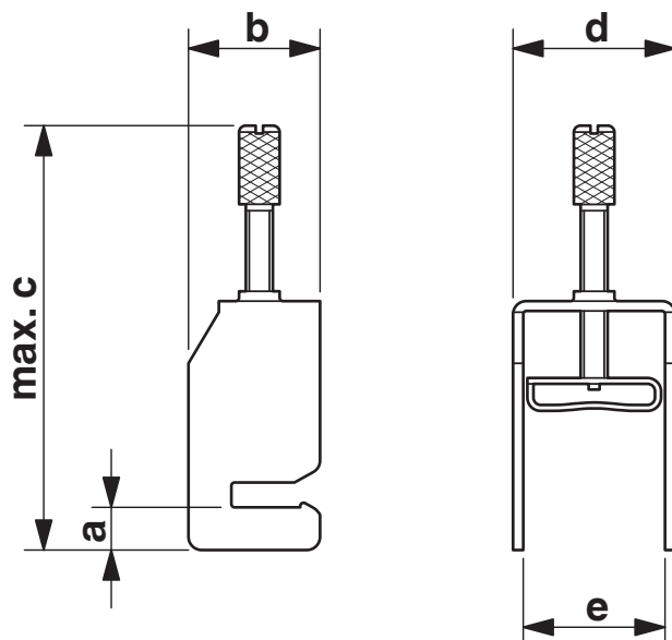
Måttskiss
