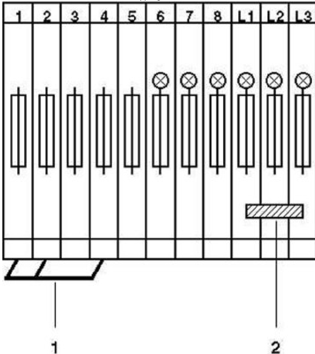
Kopplingsschema
