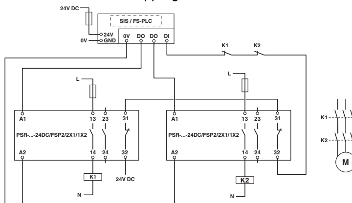
Kopplingsschema
