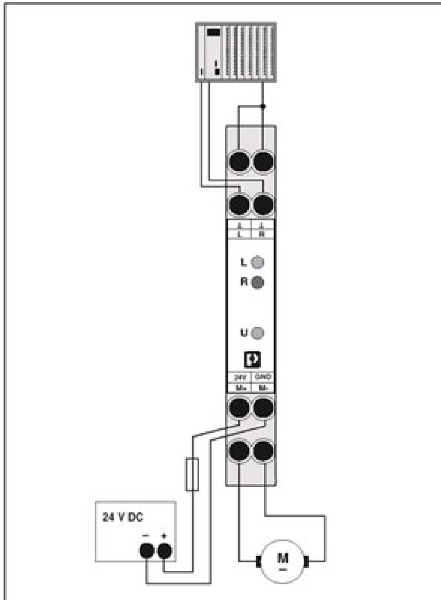
Applikationsritning
