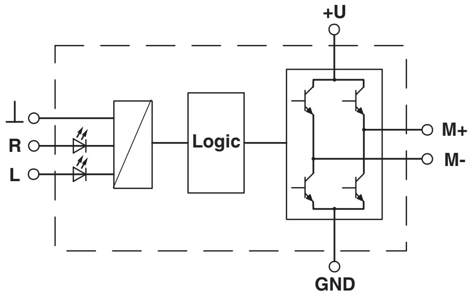
Kopplingsschema
