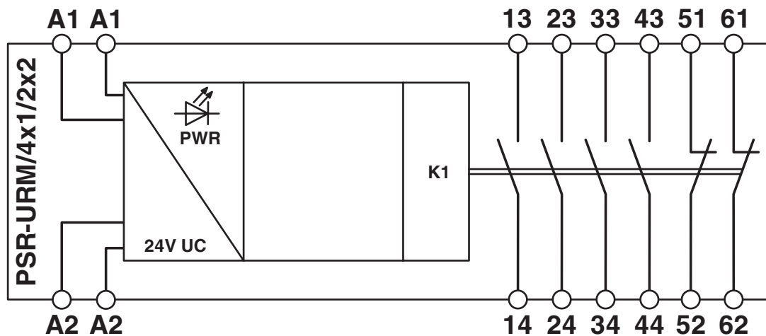
Kopplingsschema
