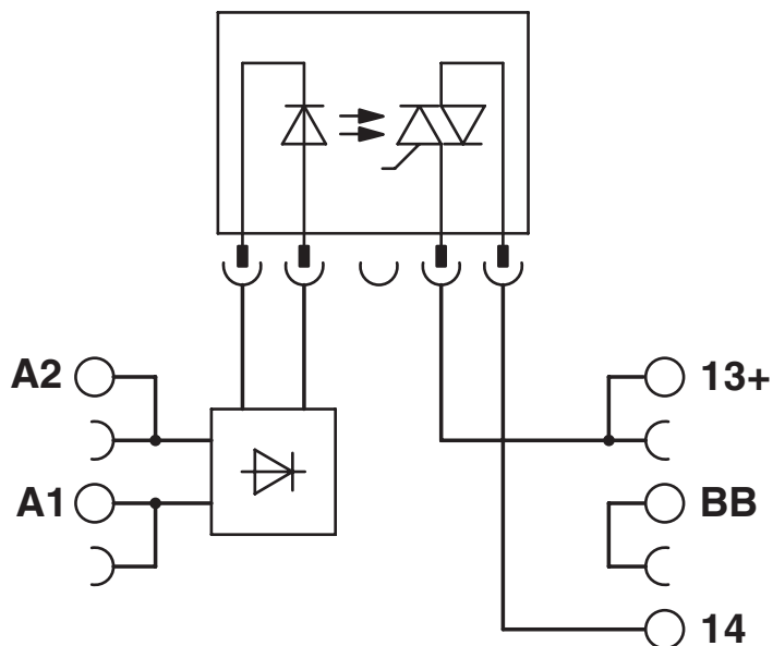
Kopplingsschema
