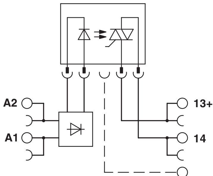
Kopplingsschema
