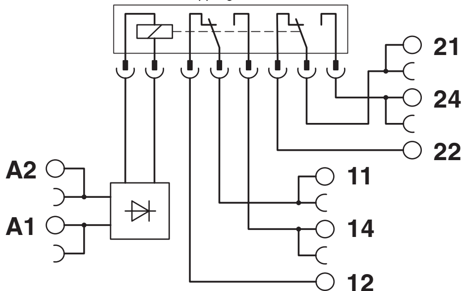
Kopplingsschema
