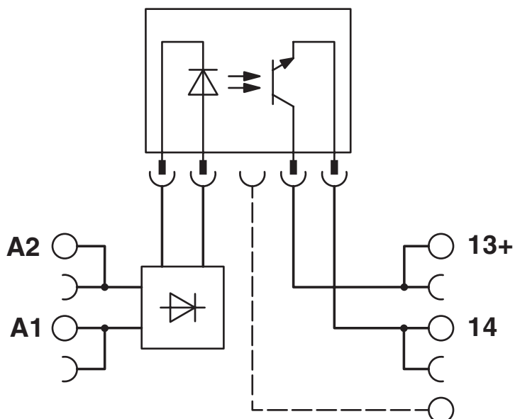
Kopplingsschema
