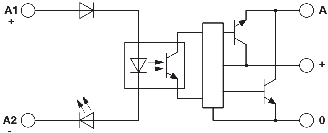
Kopplingsschema
