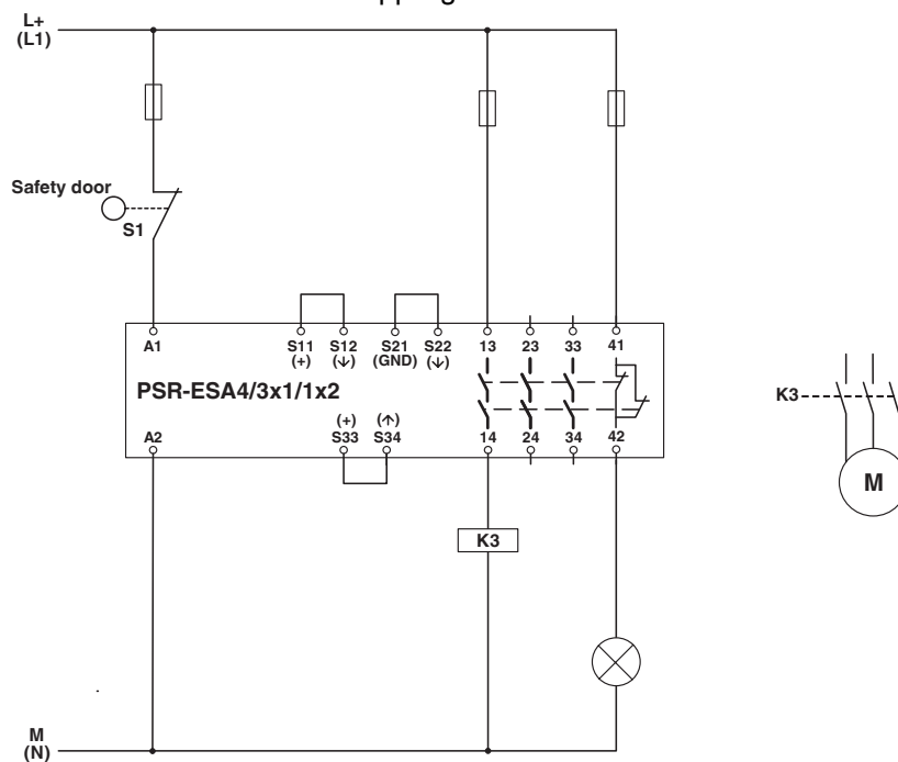
Kopplingsschema
