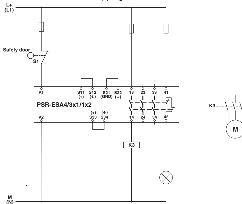
Kopplingsschema
