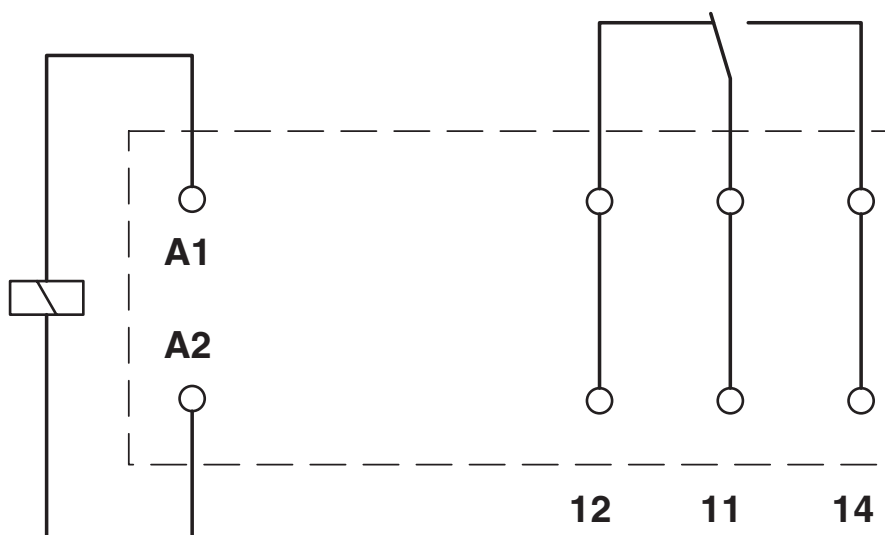
Kopplingsschema
