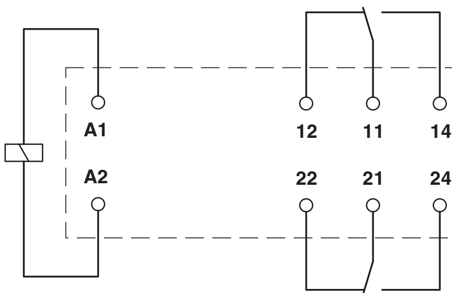
Kopplingsschema
