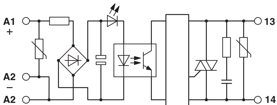
Kopplingsschema
