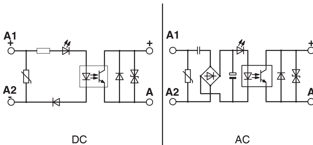
Kopplingsschema
