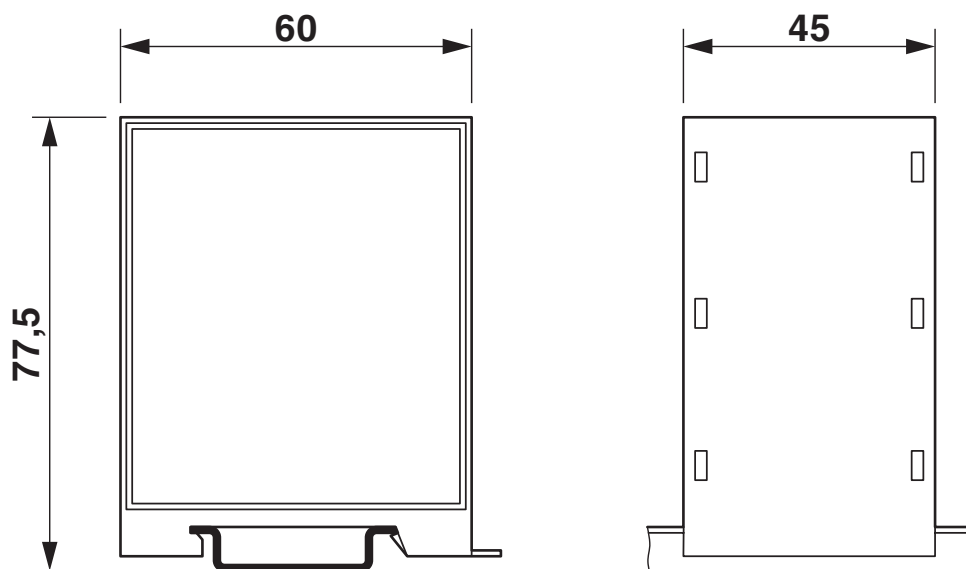
Måttskiss
