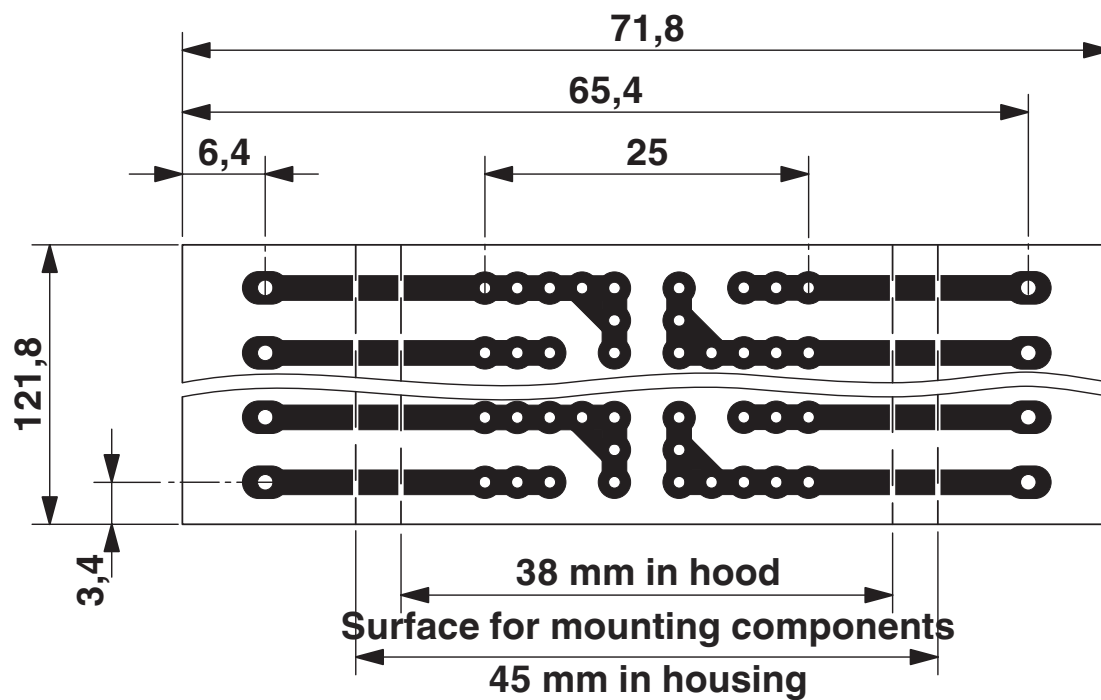
Måttskiss
