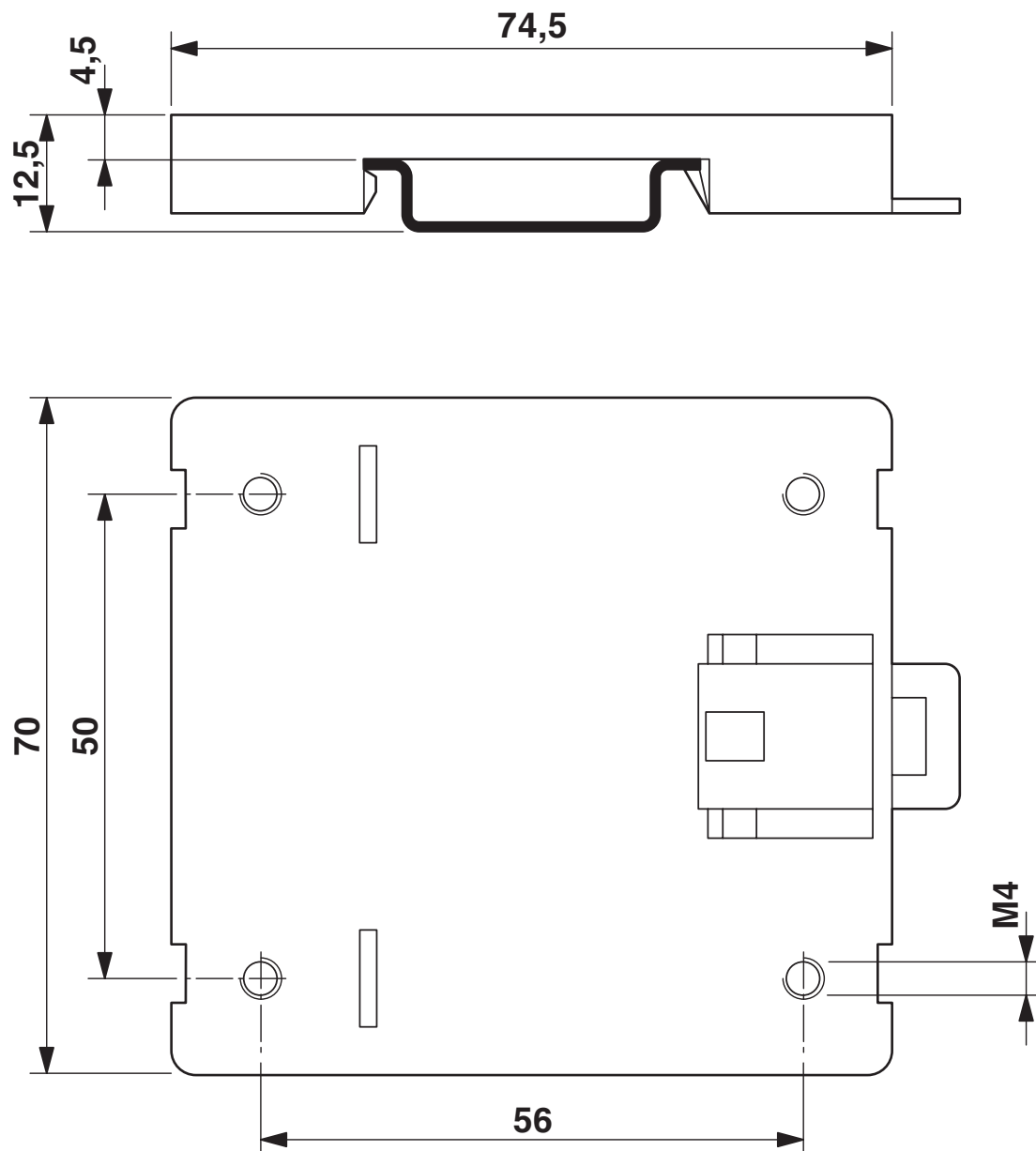
Måttskiss
