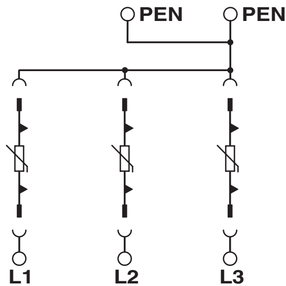
Kopplingsschema
