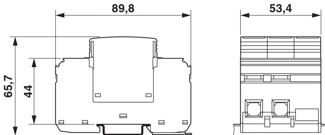
Måttskiss
