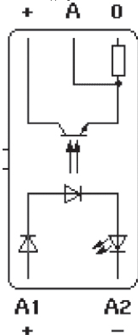
Kopplingsschema
