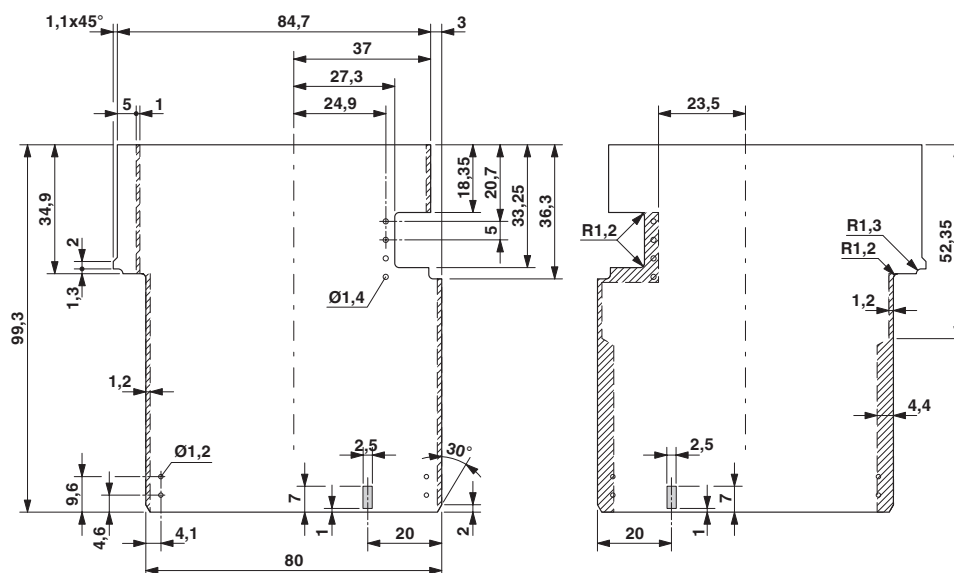
Måttskiss
