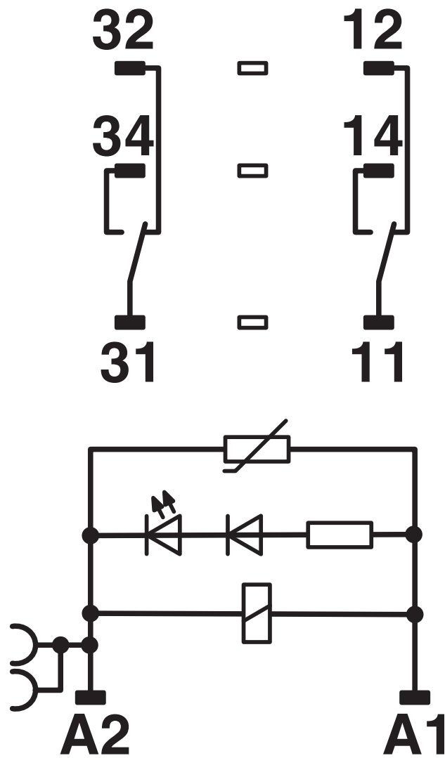
Kopplungsschema
