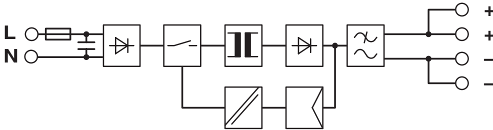
Kopplingsschema
