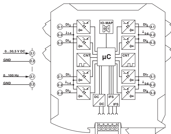
Kopplingsschema
