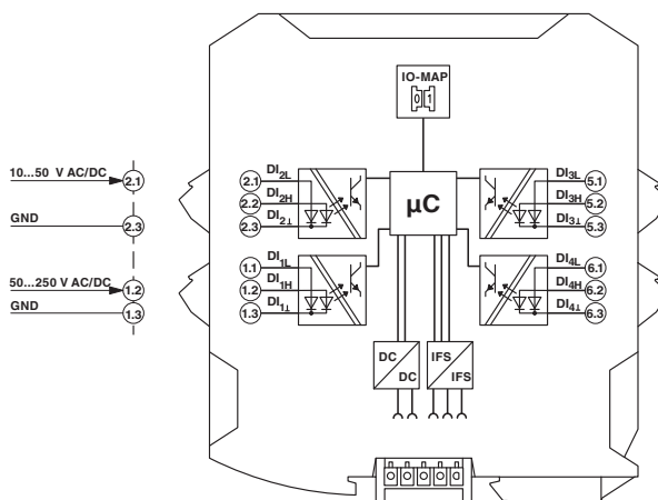
Kopplingsschema
