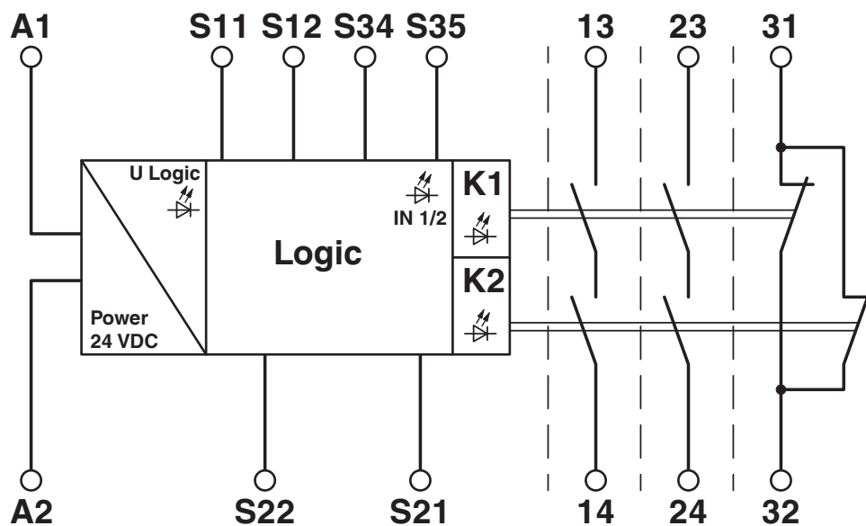
Kopplingsschema
