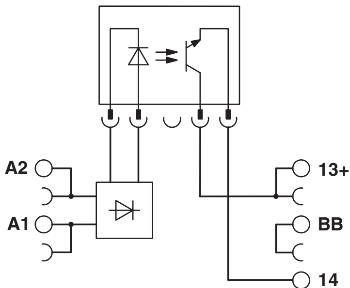
Kopplingsschema
