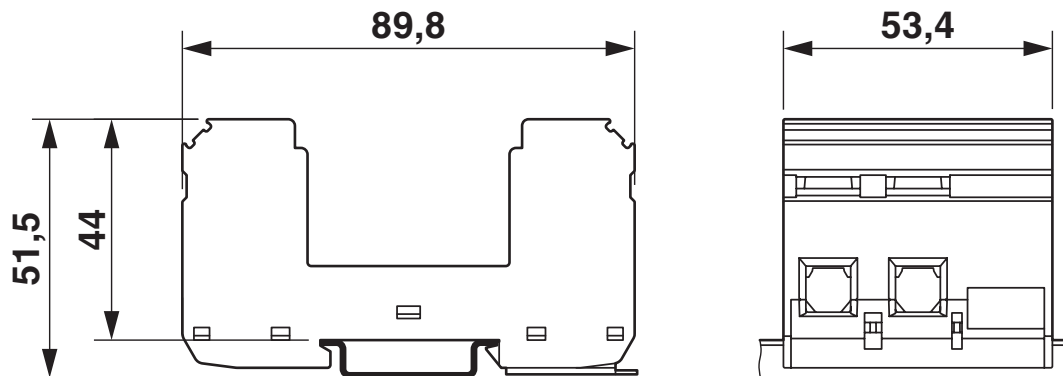
Måttskiss
