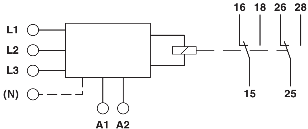
Kopplingsschema
