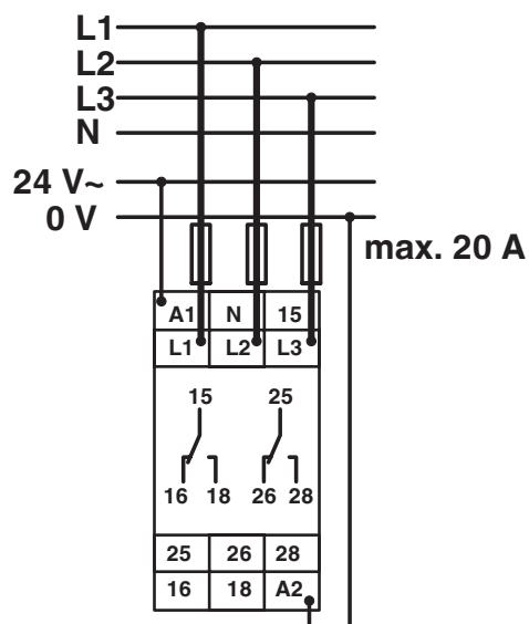
Anslutningsritning
