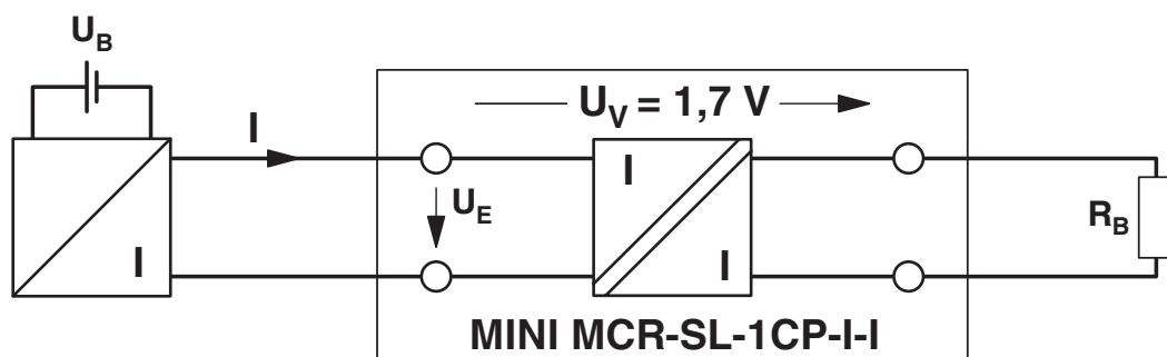
Applikationsritning
