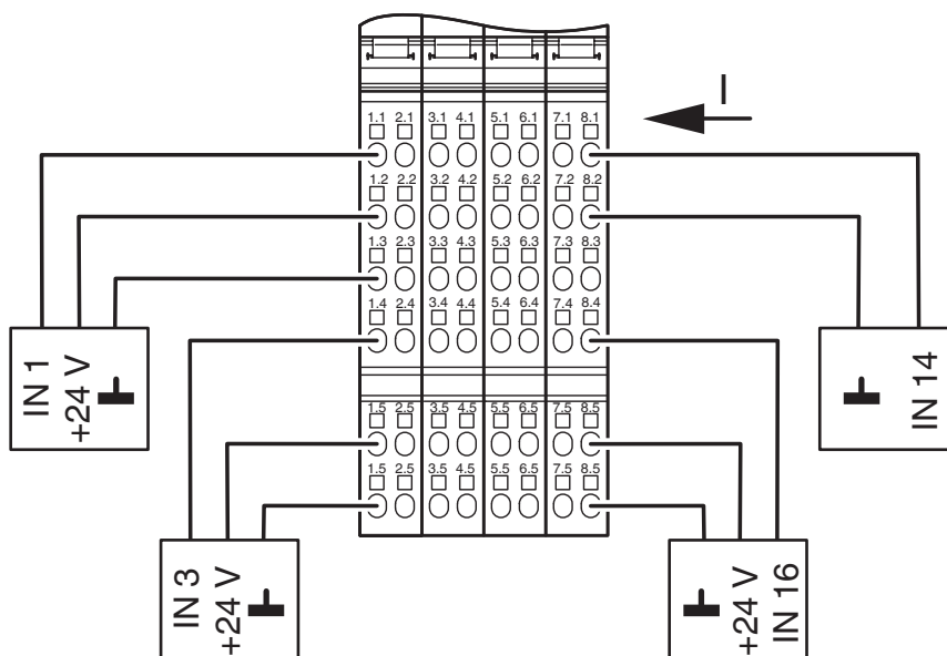
Anslutningsritning
