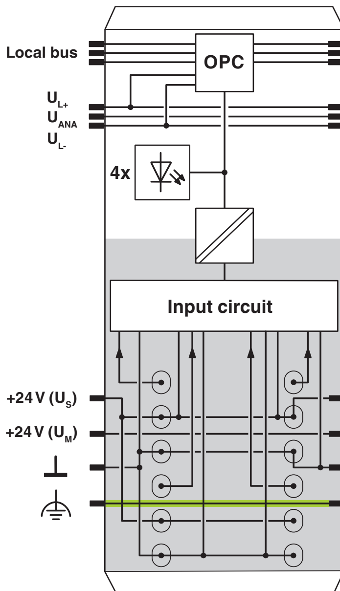
Kopplingsschema
