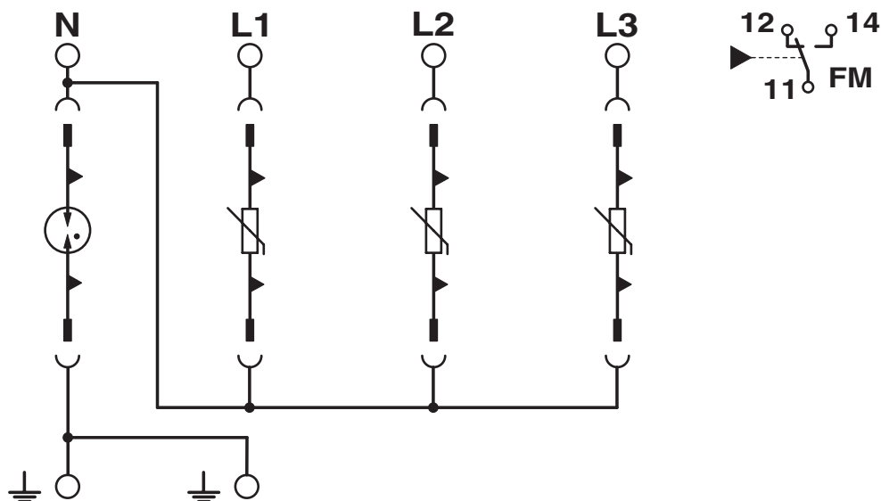
Kopplingsschema
