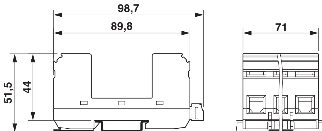
Måttskiss
