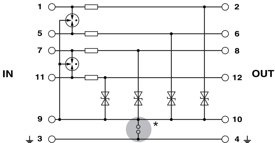
Kopplungsschema
