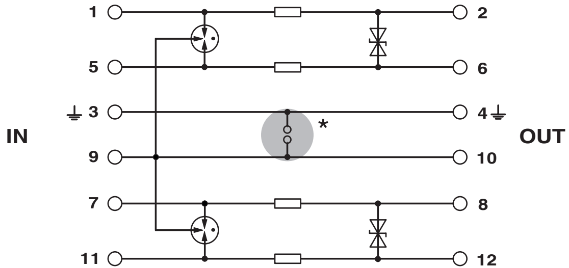
Kopplingsschema
