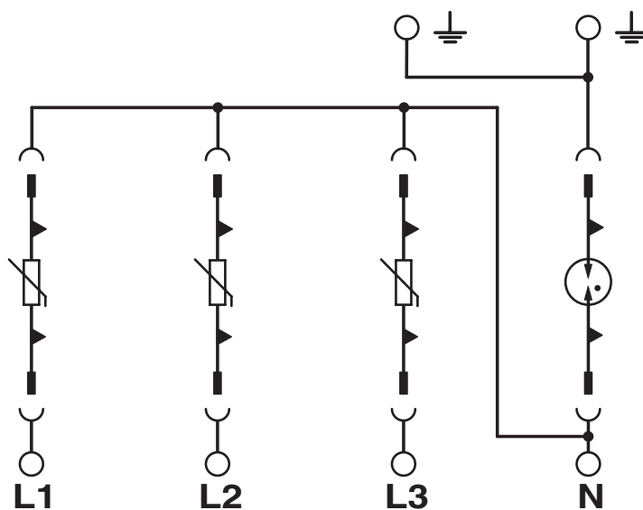
Kopplingsschema
