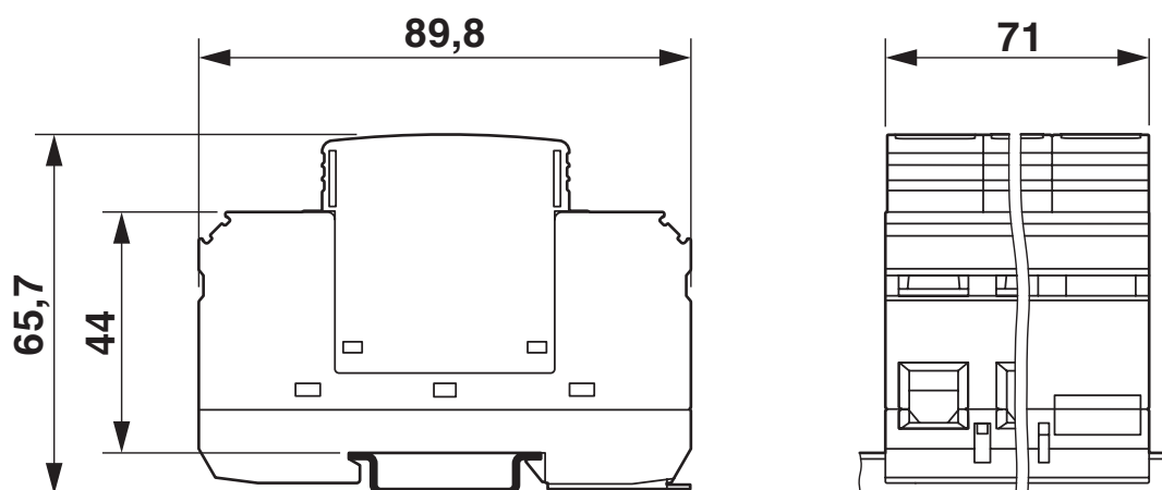
Måttskiss
