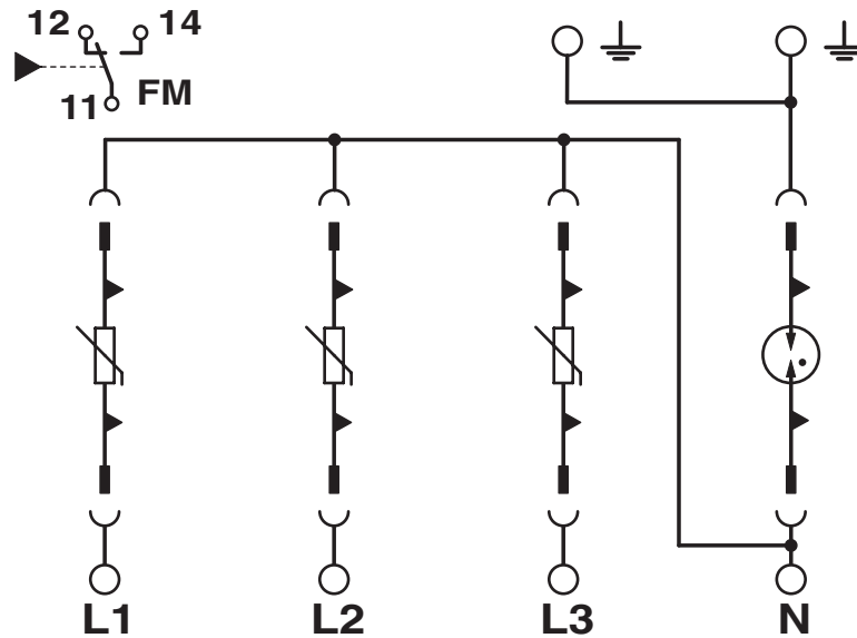
Kopplingsschema
