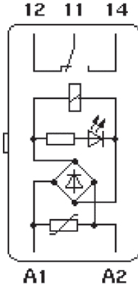
Kopplingsschema
