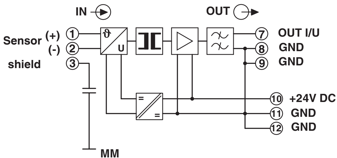
Kopplingsschema
