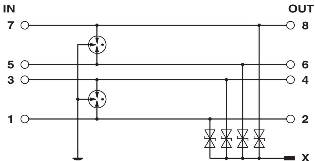
Kopplingsschema
