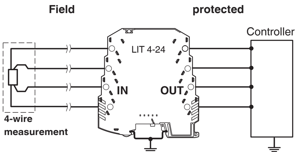
Applikationsritning
