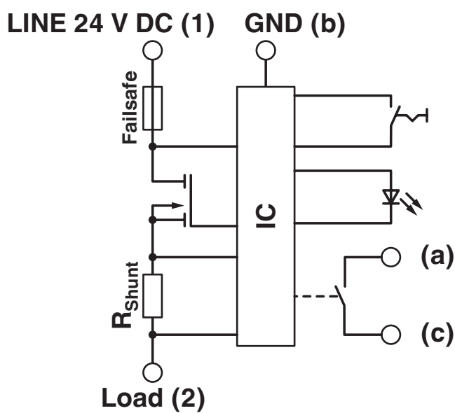
Kopplingsschema
