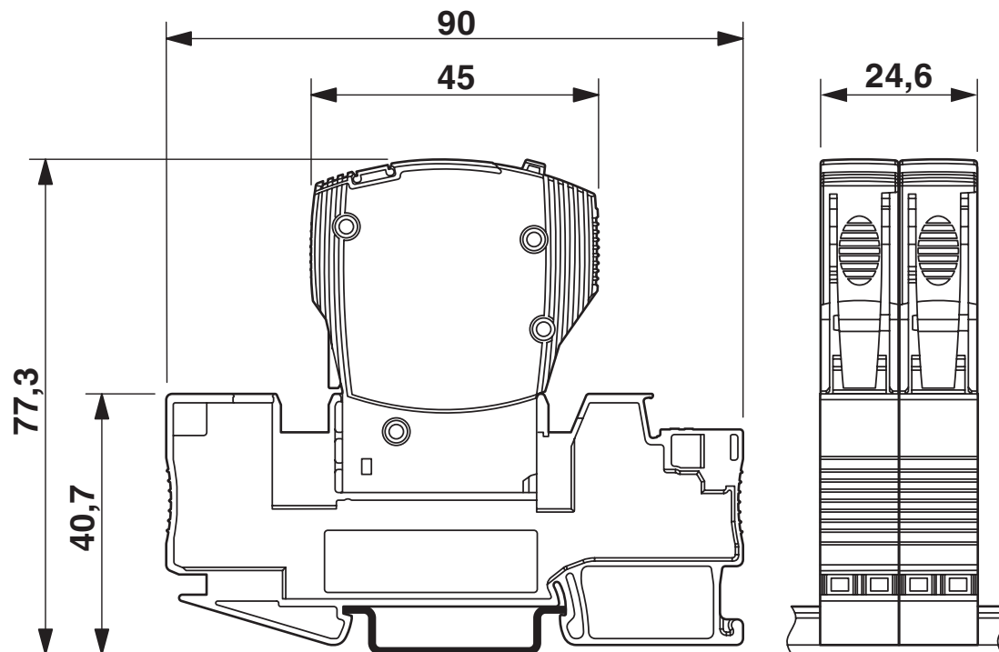
Måttskiss
