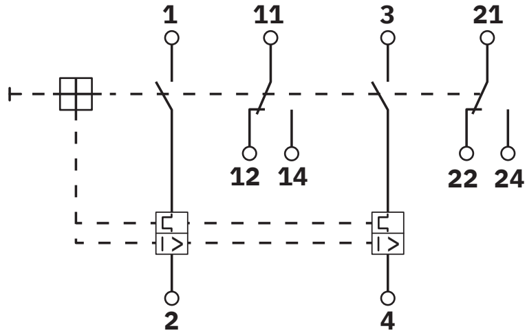
Kopplungsschema
