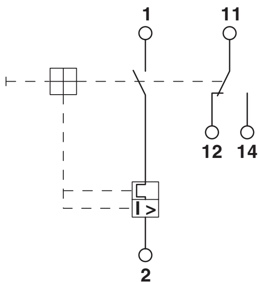
Kopplingsschema
