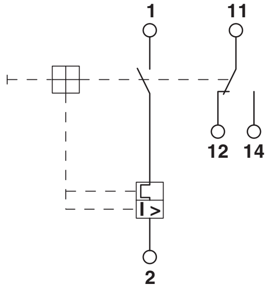
Kopplungsschema
