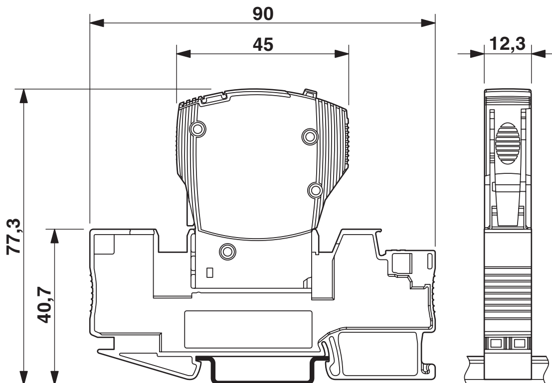
Måttskiss
